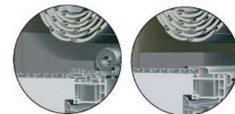
Fensteranschluss-Systeme „Click“ zum Aufrasten oder „Slide“ mit Abrollprofil
