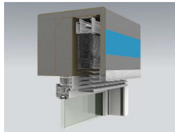
Raffstore-Aufsatzkasten System „Slide“
