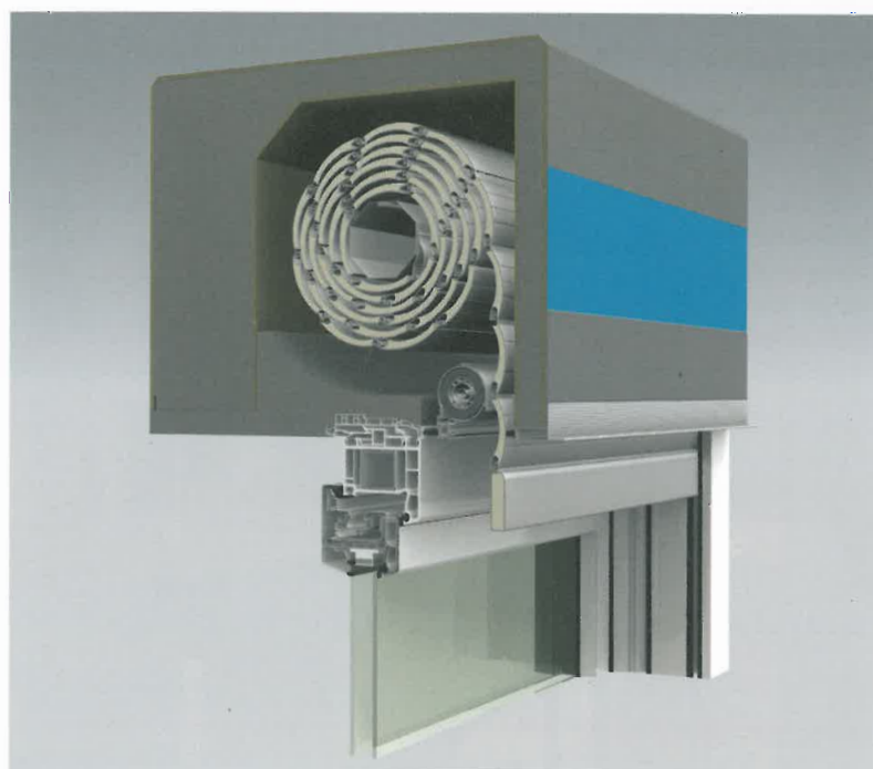
Beispiel für das Aufsatzkastensystem „Click“.
